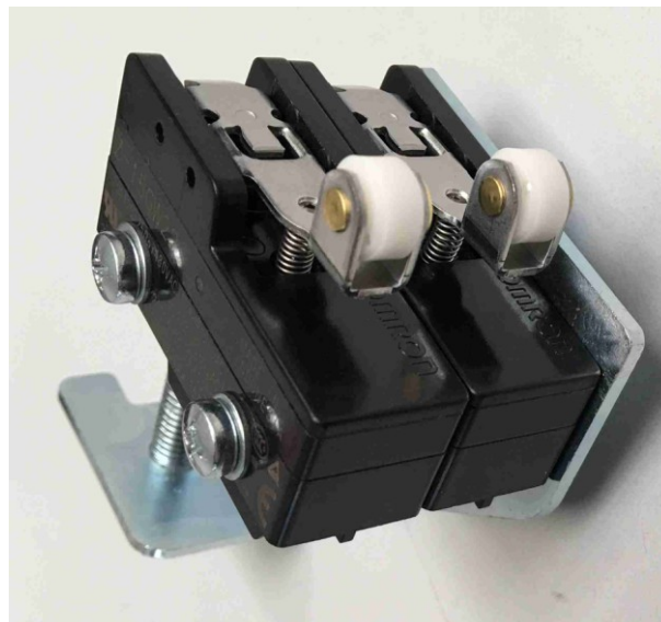
Ansicht Endschalter
